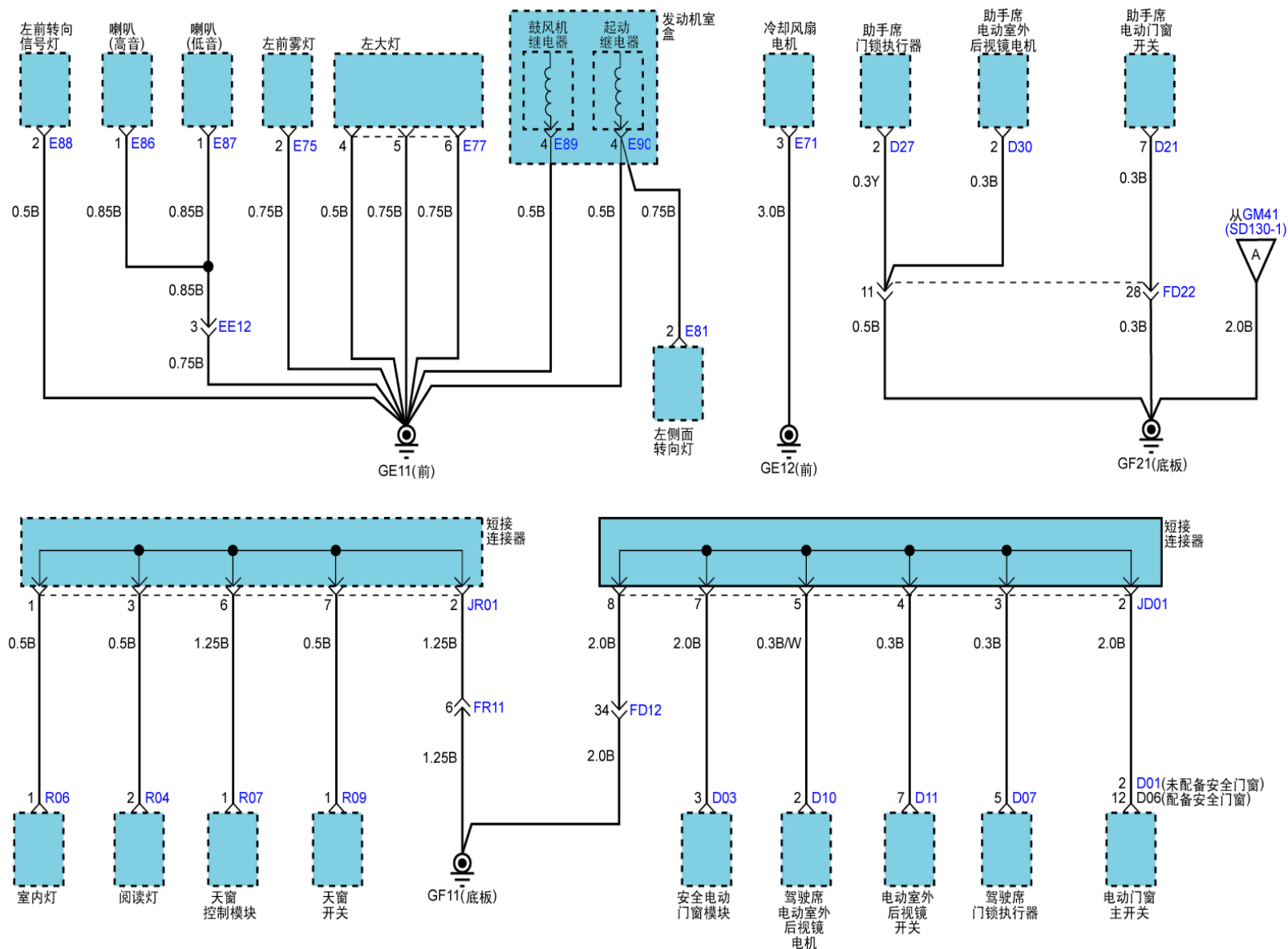
搭铁分布(2)
